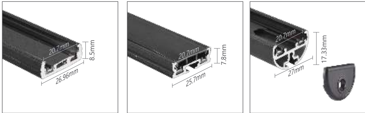
26-1 明装轨道
