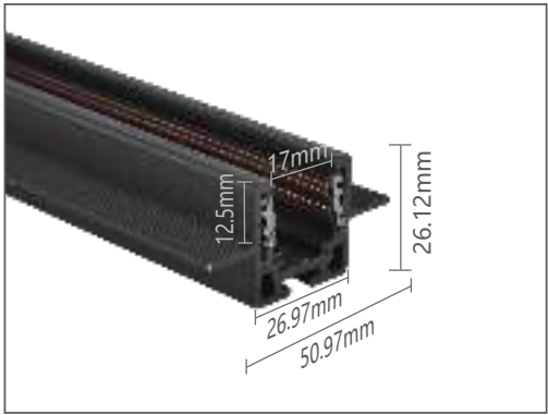
预埋圆形轨道
