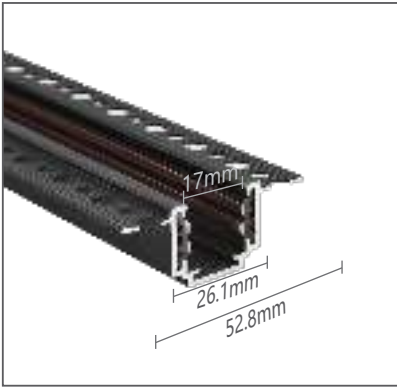
批灰轨道
