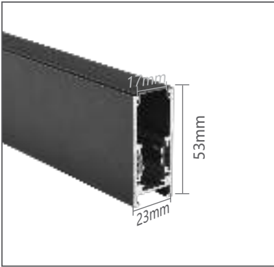
明装轨道
